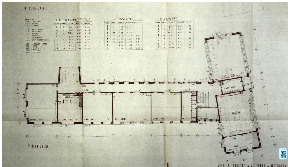
afb. 119 Plattegrond eerste verdieping 1953 (GA 9110-9135)
