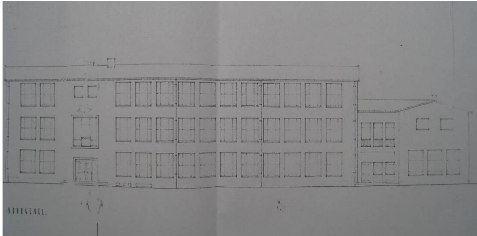
afb. 118 Voorgevel uit 1953 (GA 9110-9135)
