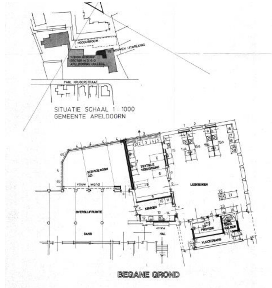
afb. 122 Uitsnede van de nieuwe toestand in 1992 (gemeente Apeldoorn)
