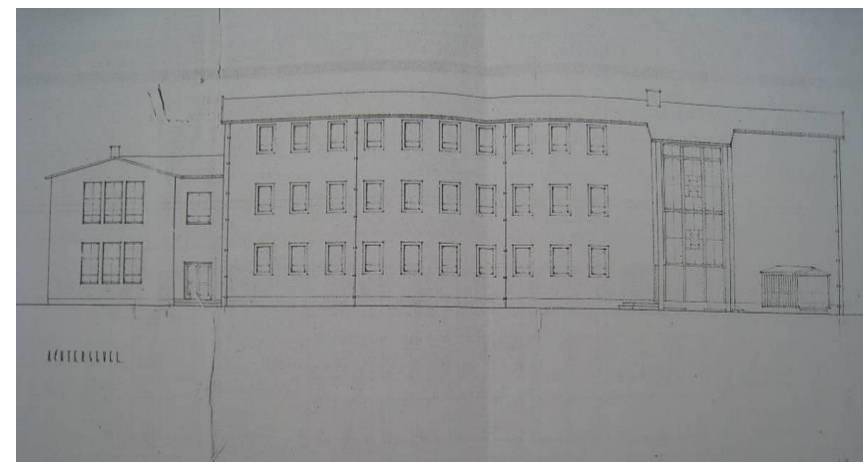
afb. 116 en 117 Linker zijgevel en achtergevel (hier nog zonder overblijflokaal) uit 1953 (GA 9110-9135)
